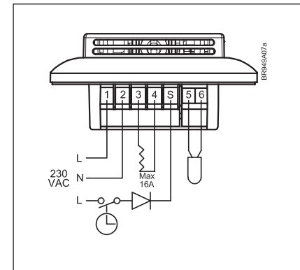
Frostschutz
