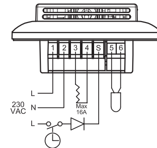
Ochrona antyzamarzaniowa
