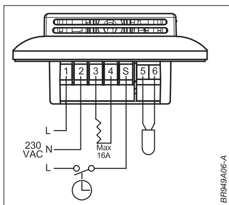
Nachtabenkung
